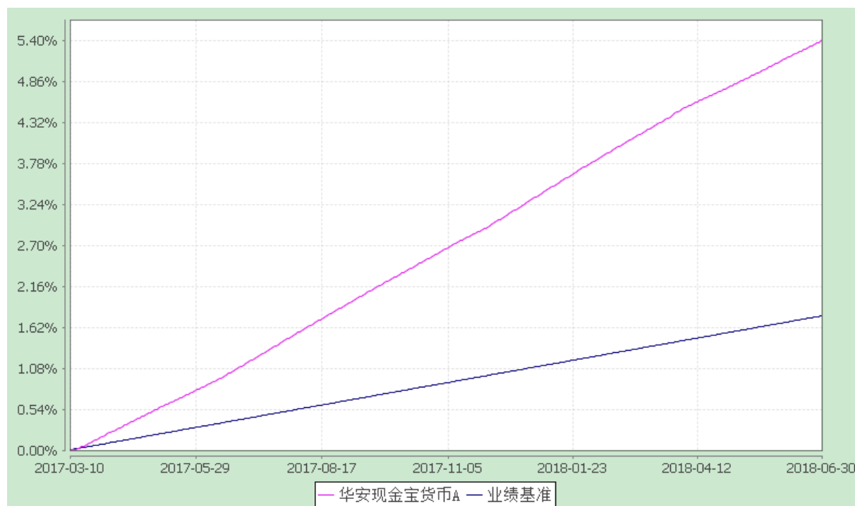
华安现金宝货币市场基金 累计净值收益率与业绩比较基准收益率历史走势对比图 (2017 年 3 月 10 日至 2018 年 6 月 30 日)
