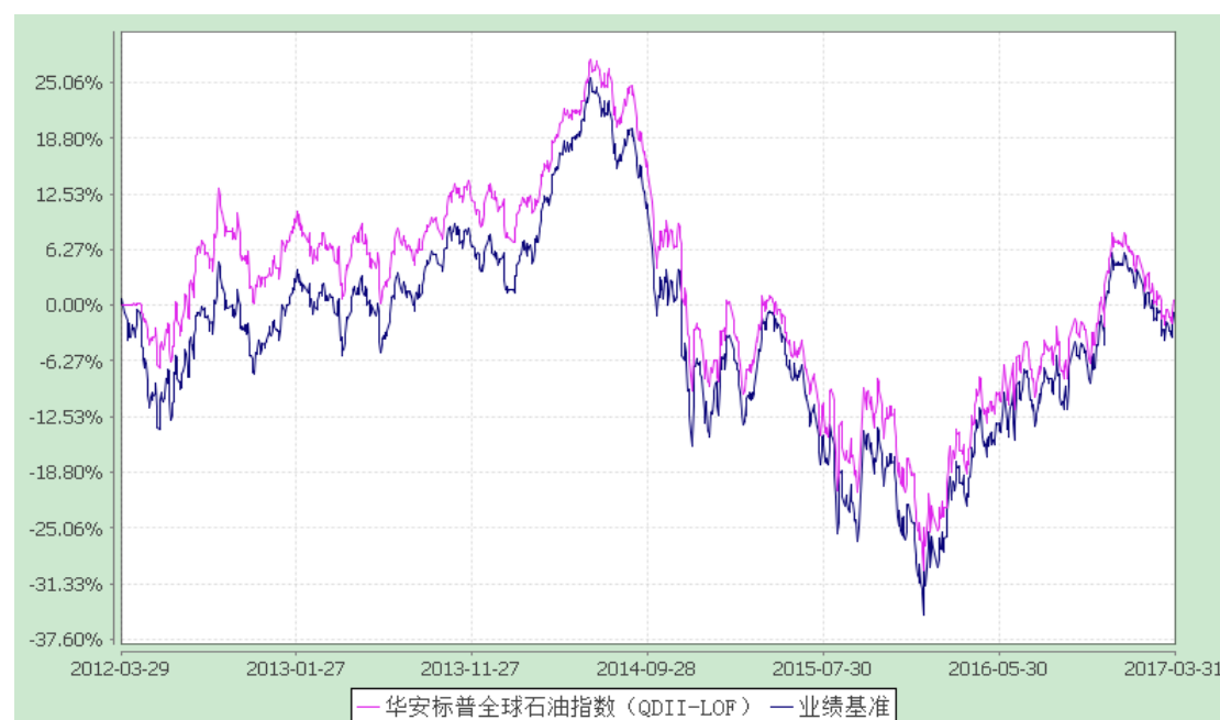
华安标普全球石油指数证券投资基金（LOF） 累计份额净值增长率与业绩比较基准收益率历史走势对比图 (2012 年 3 月 29 日至 2017 年 3 月 31 日)
